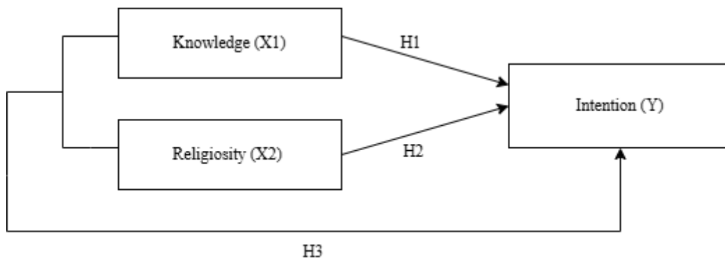
Gambar 1. Kerangka Hipotesis
